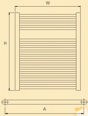
EMAS DÜZ BEYAZ BOYALI / KROM KAPLI HAVLUPAN TEKNİK ÖZELLİKLER TABLOSU
