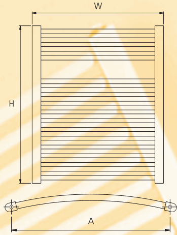
EMAS BOMBELİ BEYAZ BOYALI / KROM KAPLI HAVLUPAN TEKNİK ÖZELLİKLER TABLOSU
